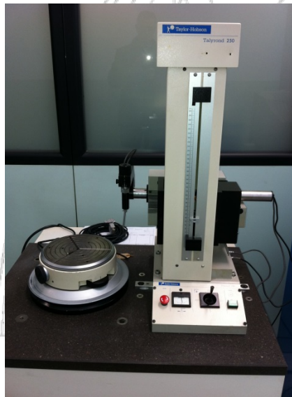
Máquina error de forma Taylor Hobson
